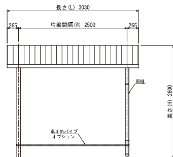
立面図
