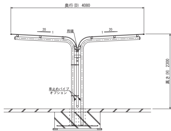
断面図
