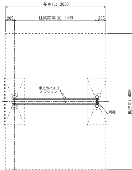
平面図
