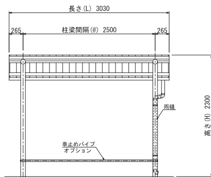
立面図
