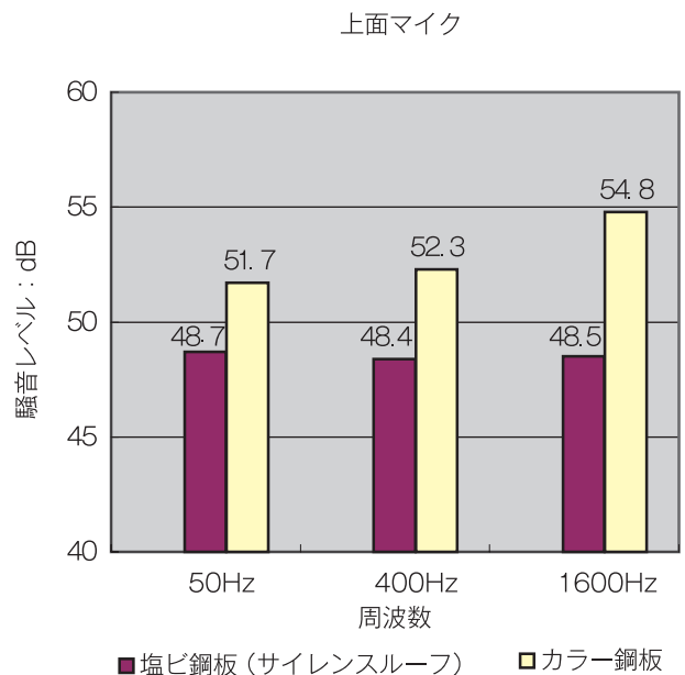
屋根材の降雨時発生騒音試験の結果
