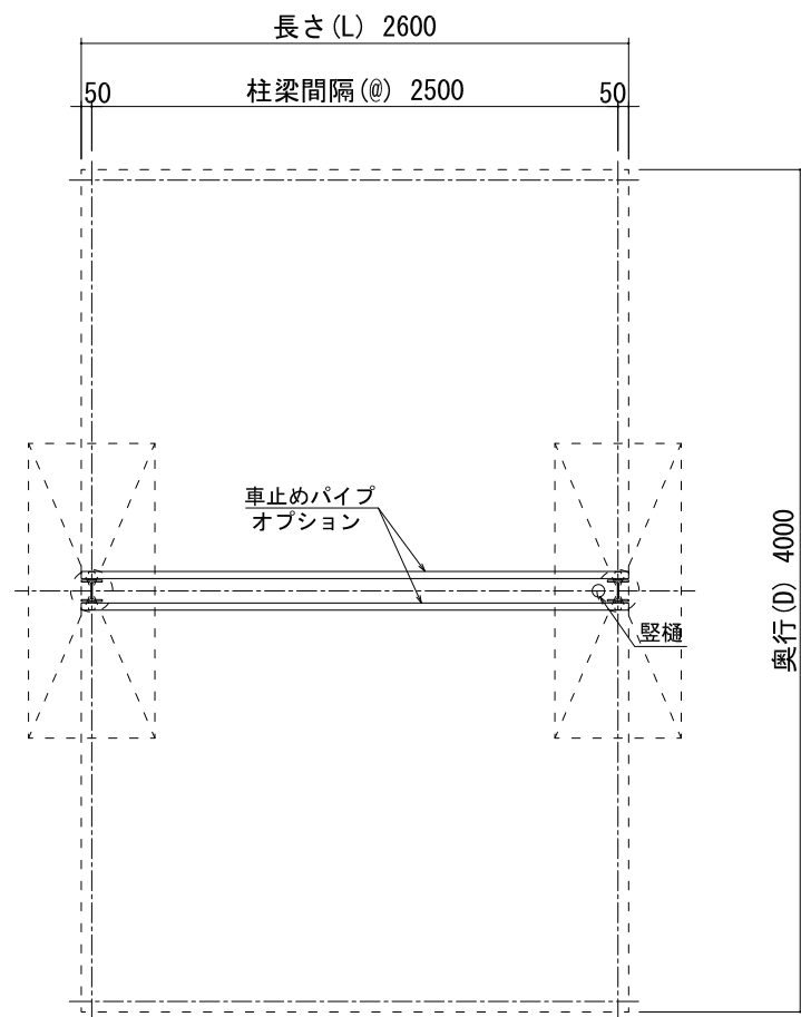
平面図
