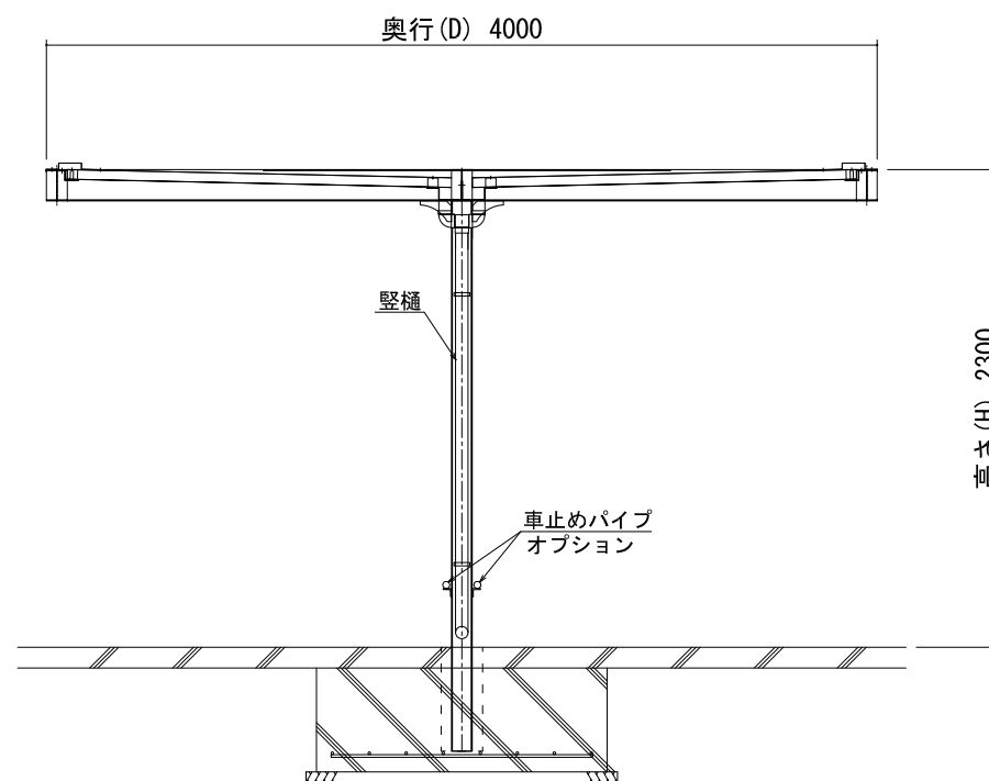
断面図
