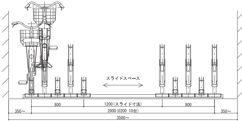
立面図
