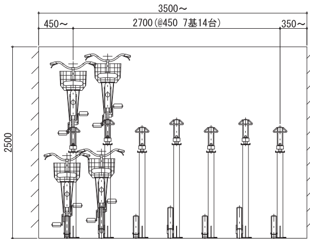
立面図
