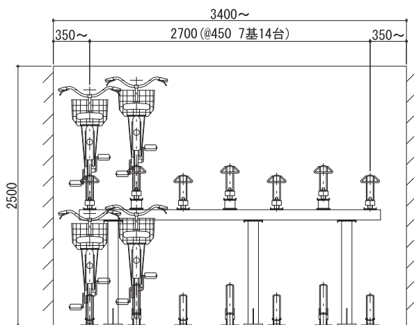
立面図
