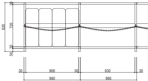
正面詳細図
