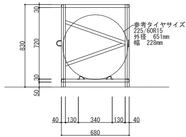
側面断面図
