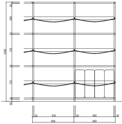
正面詳細図
