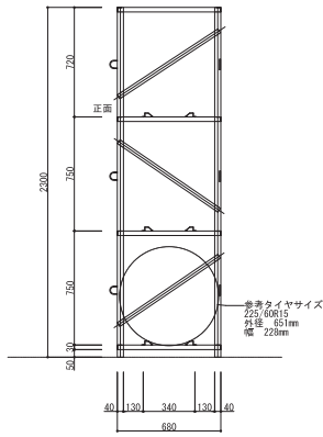
側面断面図
