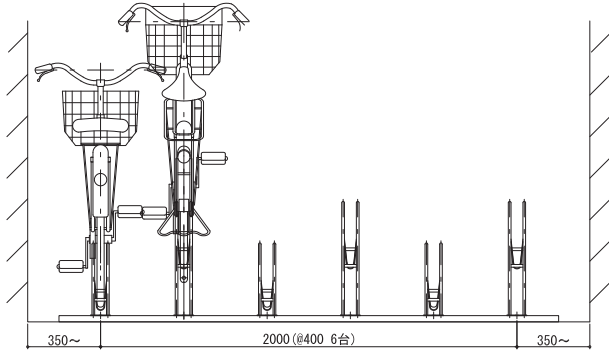
立面図
