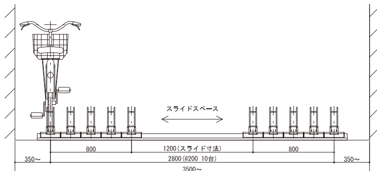
立面図
