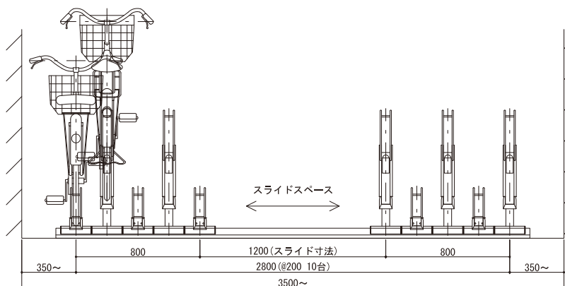
立面図
