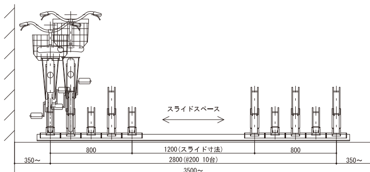
立面図
