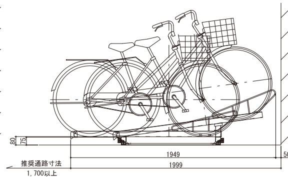
断面図
