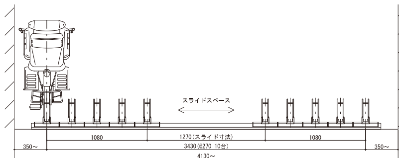
立面図
