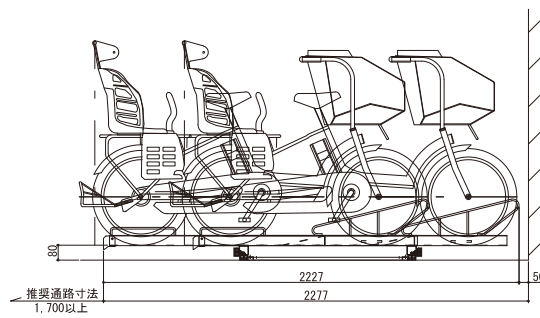
断面図
